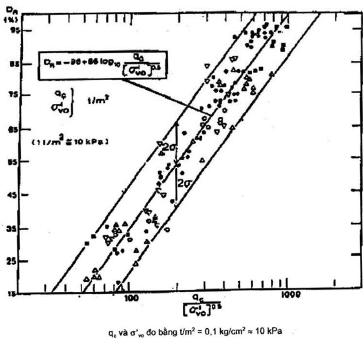
Hình VI-7: D của đất có kết bình thường (Jamolkowsky và cộng sự 1995).
