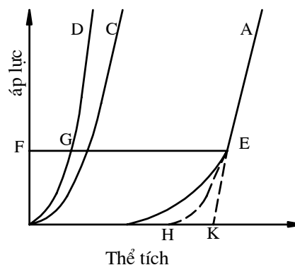
Hình VI-14: Đường hiệu chỉnh thể tích
