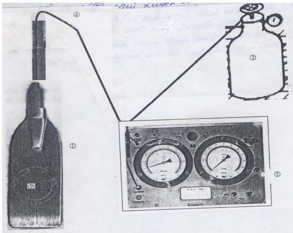
Hình VI-16: Sơ đồ của thí nghiệm: 1) mũi xuyên phẳng; 2) màng thép; 3) bình khí; 4) dây cáp dẫn khí nén; 5) hộp điều khiển; 6) cân xuyên
