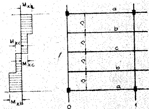
Hình 6-20. Sơ đồ vị trí các dầm và biểu đồ mômen xoắn trong trường hợp ba dầm giữa.
