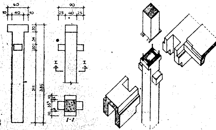
Hình 1-4. Cột được nối tại chỗ có mômen bằng không (khớp). Nối cột bằng thép bản đặt sẵn khi đúc cột và khi lắp xong thì vận các bulông lại. Dầm chữ U được gối lên tại cột và ôm chặt chỗ liên kết ở hai đầu cột.
