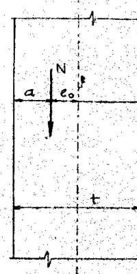
Hình 6-12. Mặt cắt của vách cứng thẳng đứng.
