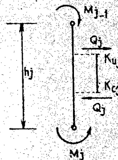
Hình 2-8. Sơ đồ để xác định lực cắt tổng thể của vách cứng tổng thể.
