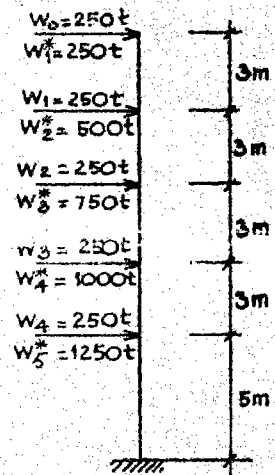
Hình 5-3. Tải trọng nằm ngang của hệ thay thế.
