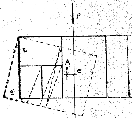
Hình 6-23. Ngoại lực P tác dụng lệch tâm.
