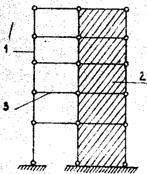
Hình 1-2. Sơ đồ kết cấu của nhà khung khớp (mặt cắt đứng ngang nhà): 1 - hệ khung khớp (cột-dầm-giằng); 2 - vách cứng thẳng đứng; 3 - vách cứng nằm ngang.
