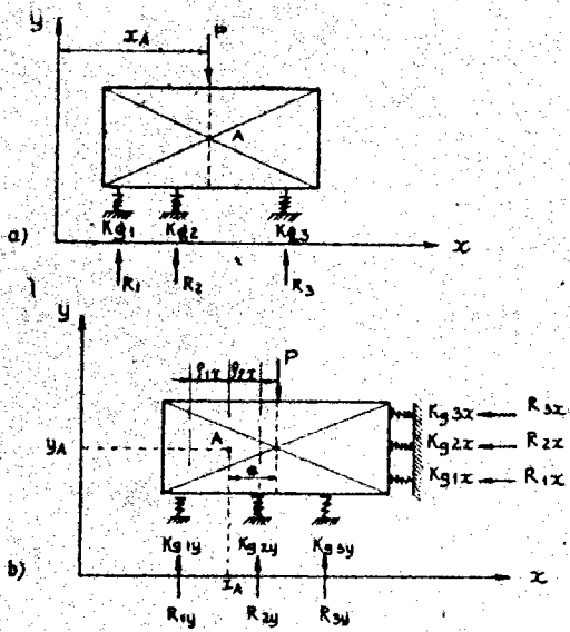
Hình 6-7. Phân bố tải trọng nằm ngang lên các vách cứng thẳng đứng: a) trường hợp lực P đi qua tâm xoắn A ; b) trường hợp lực P không đi qua tâm xoắn A .
